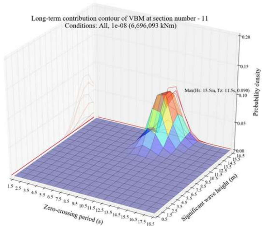
그림 2.1 종급힘모멘트의 장기해석하중에 대한 기여도 선도
