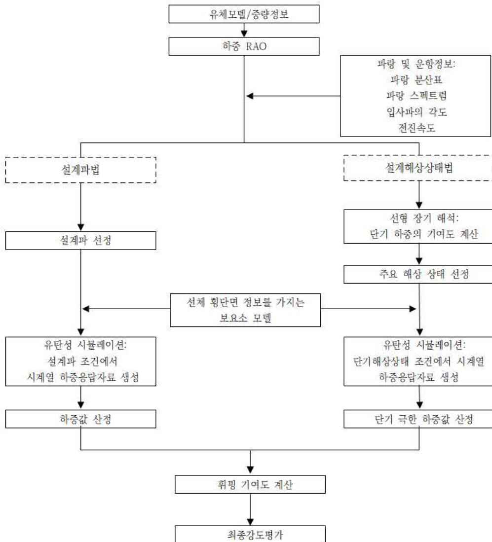
그림 1.1 휘핑영향을 고려한 선체강도 평가 절차
