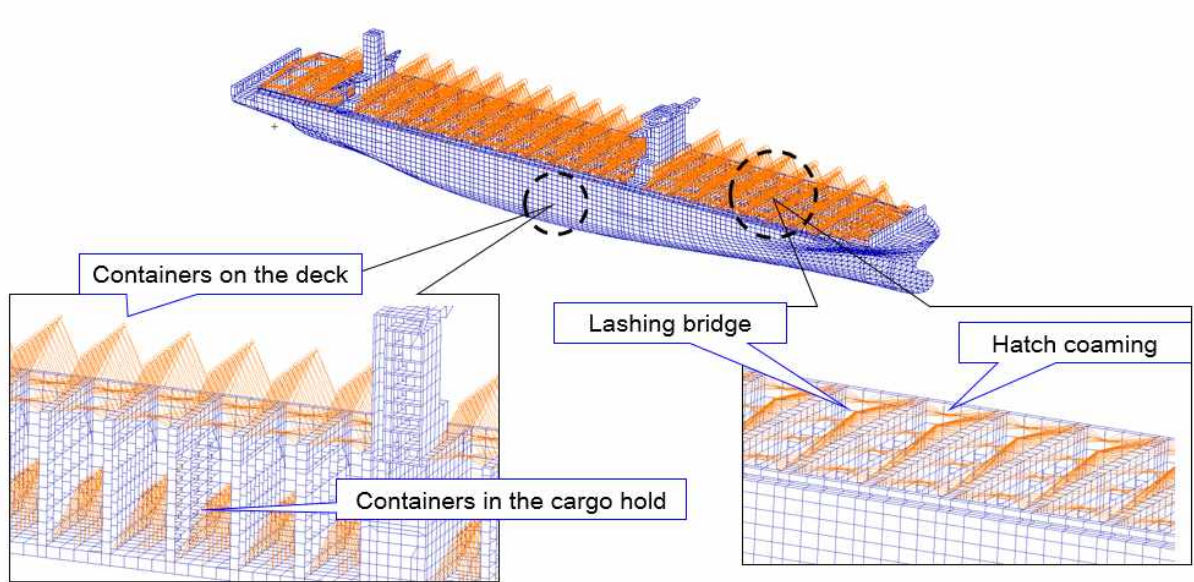
그림 3.2 질량모델을 적용한 컨테이너선의 3차원 구조해석 모델 예
